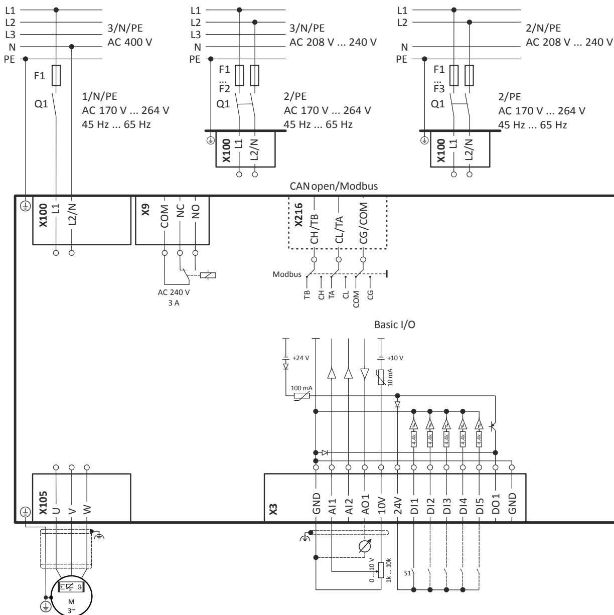
Fig. 3: Wiring example
