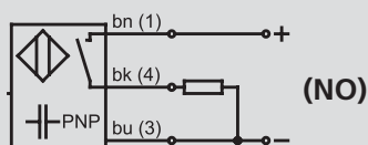
Anschlussdiagramme Connection diagrams
